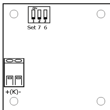
Рисунок 2. Внешний вид платы кнопки вызова MP-433W9
