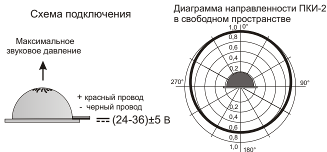
Рис.2 Схема подключения и диаграмма направленности оповещателя ПКИ-2.
