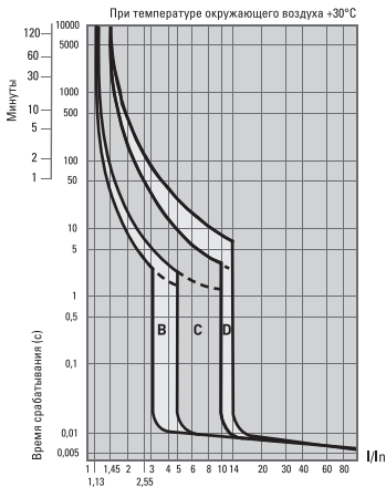
Рис. 1. Время-токовые характеристики
