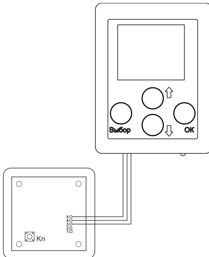
Рисунок 6. Подключение тестера к радиокнопке для установки ее номера
