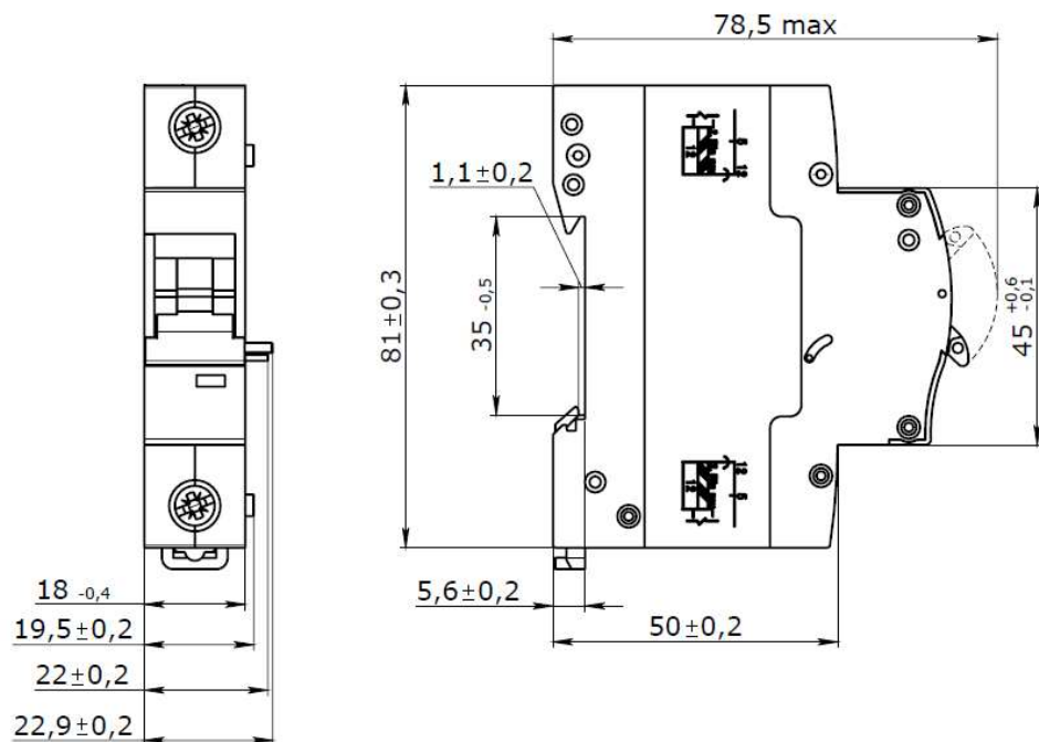
Рисунок 1.1 - Габаритные размеры SHT, UVT
