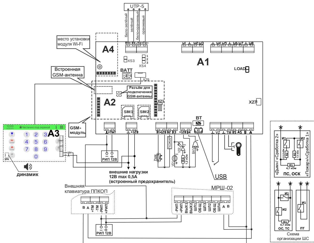
Рисунок 42 – Схема подключения прибора Приток-А-КОП-02.6
