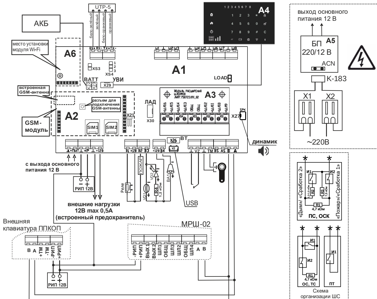
Рисунок 48 – Схема подключения прибора Приток-А-КОП-05
