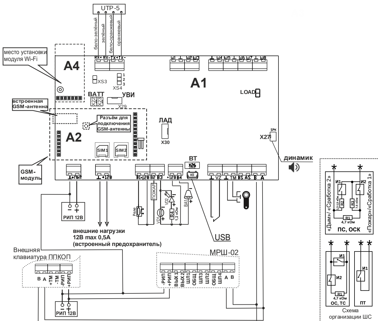
Рисунок 46 – Схема подключения прибора Приток-А-КОП-04 (D)
