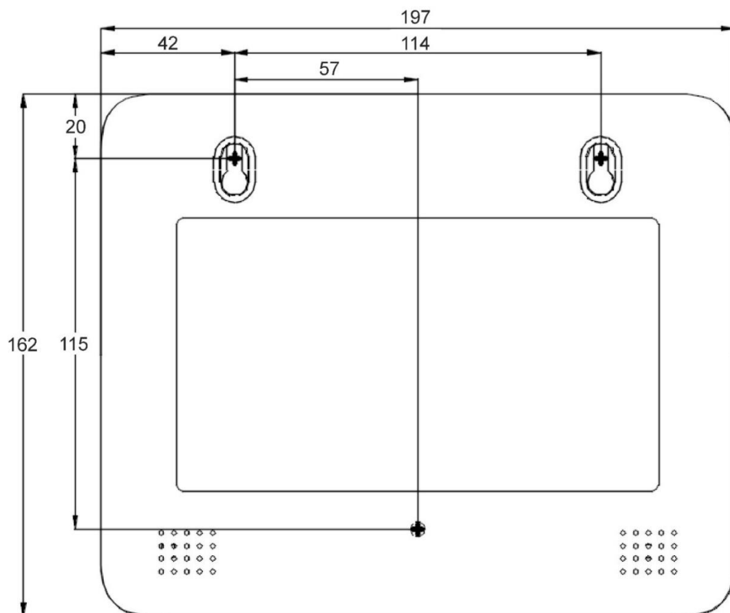
Рисунок 56 – Разметка отверстий для крепления прибора КОП-02.6, КОП-01(8), КОП-01 исп.1 и КОП-04 (вид со стороны передней панели)
