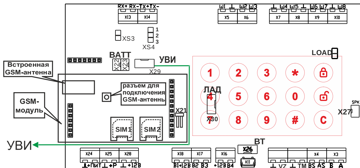
Рисунок 45 – Рекомендуемая укладка кабеля между УВИ и платой прибора
