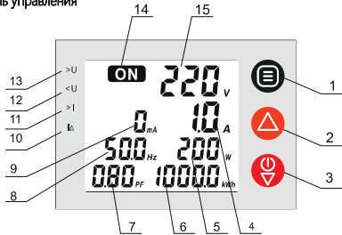
Рисунок 1 – Панель управления DPVA
