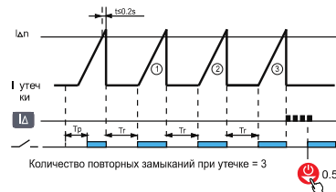
Рисунок 9 – Функциональная диаграмма тока утечки реле DPVA Когда ток утечки в цепи превысит установленное значение, устройство защиты отключится. Вы можете отключить функцию защиты от утечки. Данный фильтр будет сброшен в соответствии с заданным
