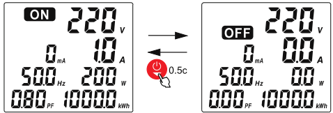
Рисунок 2 – Внешний вид панели при ручном включении реле DPVA
