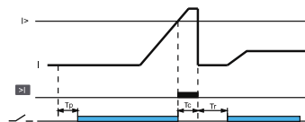
Рисунок 8 – Функциональная диаграмма перегрузки по току реле DPVA Когда текущее значение превысит установленное значение тока и продлится в течение времени Td, защита выключится и начнет сброс с задержкой Tr. По истечении времени сброса она снова включится.
