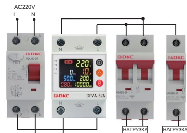
Рисунок 6 – Схема подключения реле DPVA
