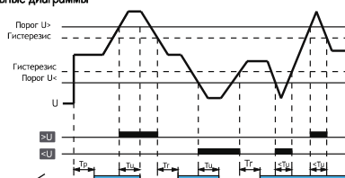
Рисунок 7 – Функциональная диаграмма перенапряжения и понижения напряжения реле DPVA При возникновении ошибки перенапряжения/пониженного напряжения устройство защиты выключится. Когда напряжение вернется в норму, устройство защиты включится через время сброса, а значение перенапряжения/пониженного напряжения может быть заново установлено.
