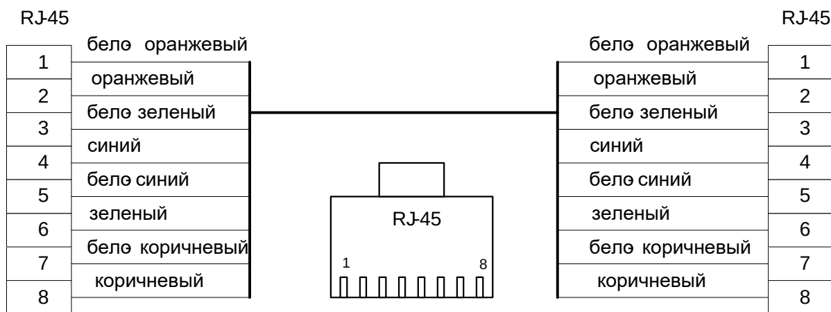
Рис. 6.4. Разделка кабеля.
