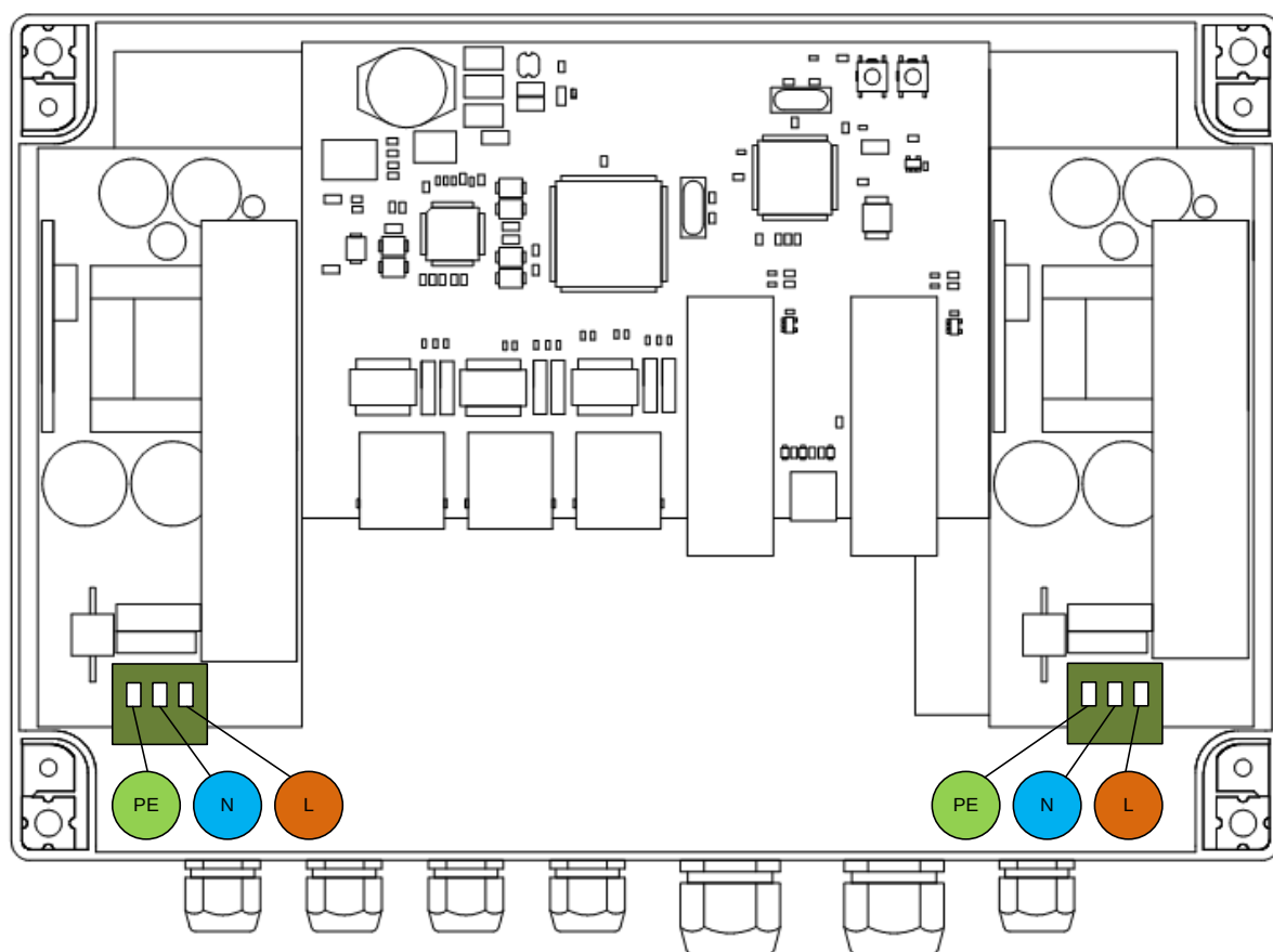
Рис. 6.3-1. Подключение питания к PSW-1G4F.
