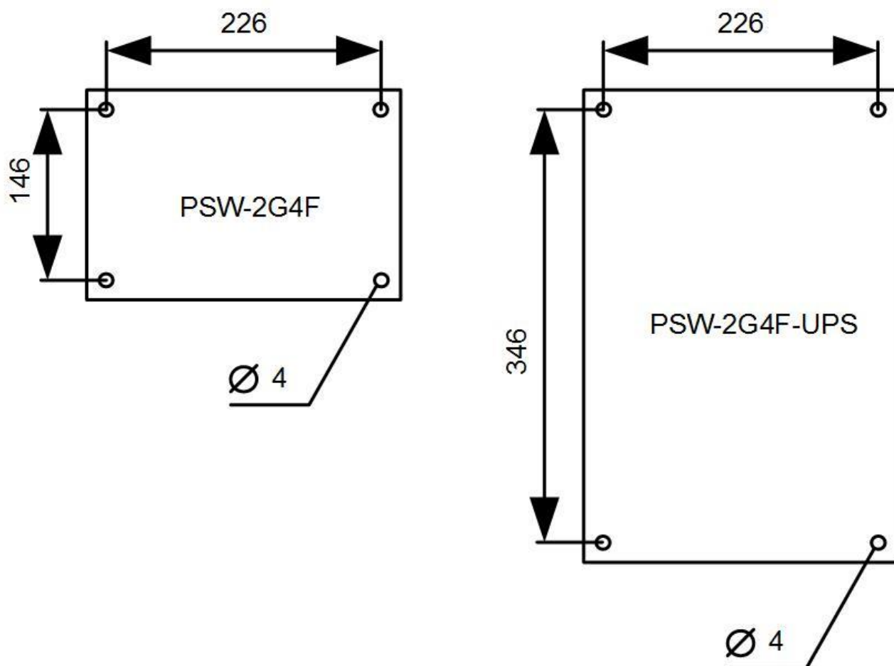
Рис. 6.1.1. Разметка крепления
