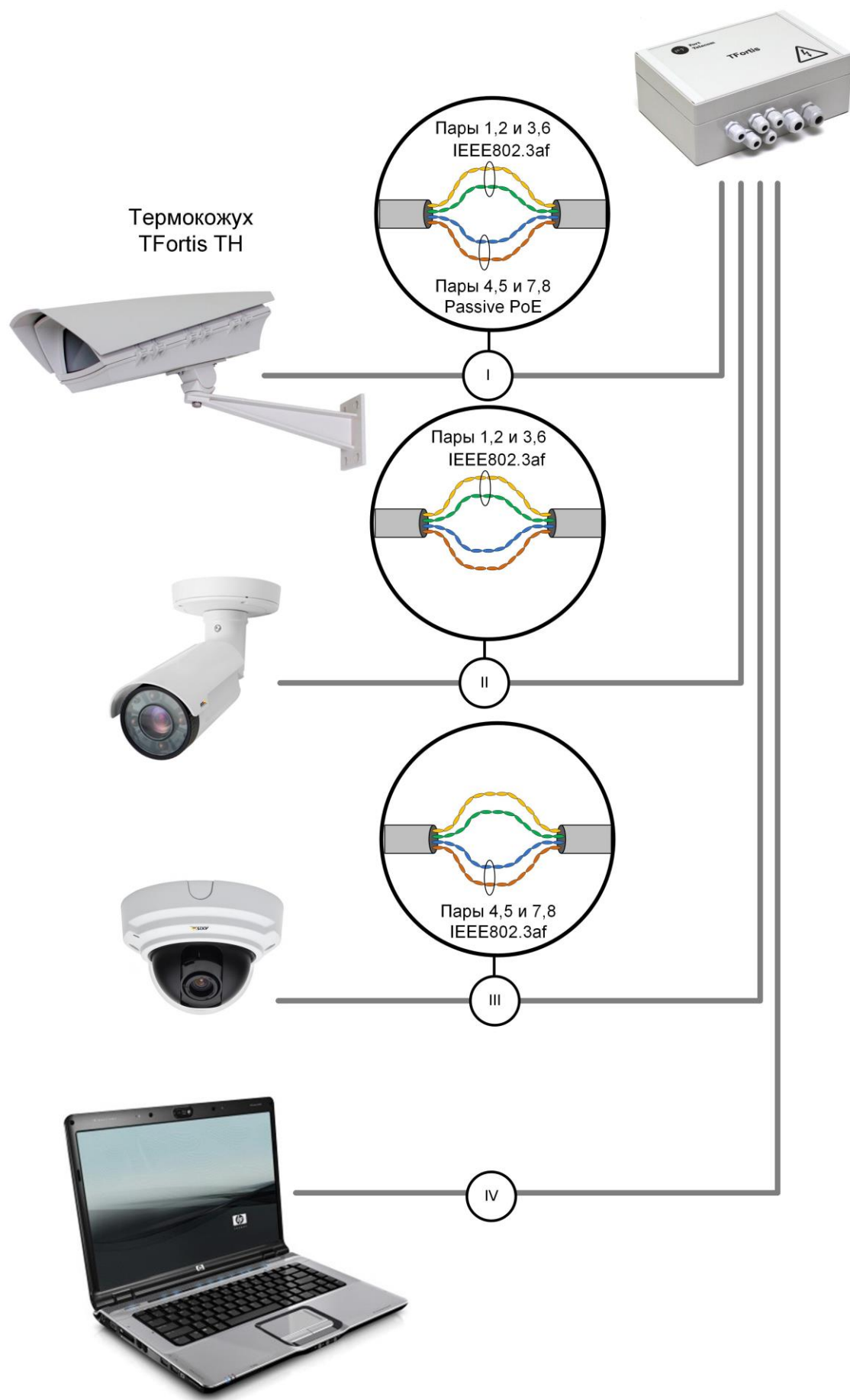
Рис. 2.3. Схема питания по PoE для разных случаев
