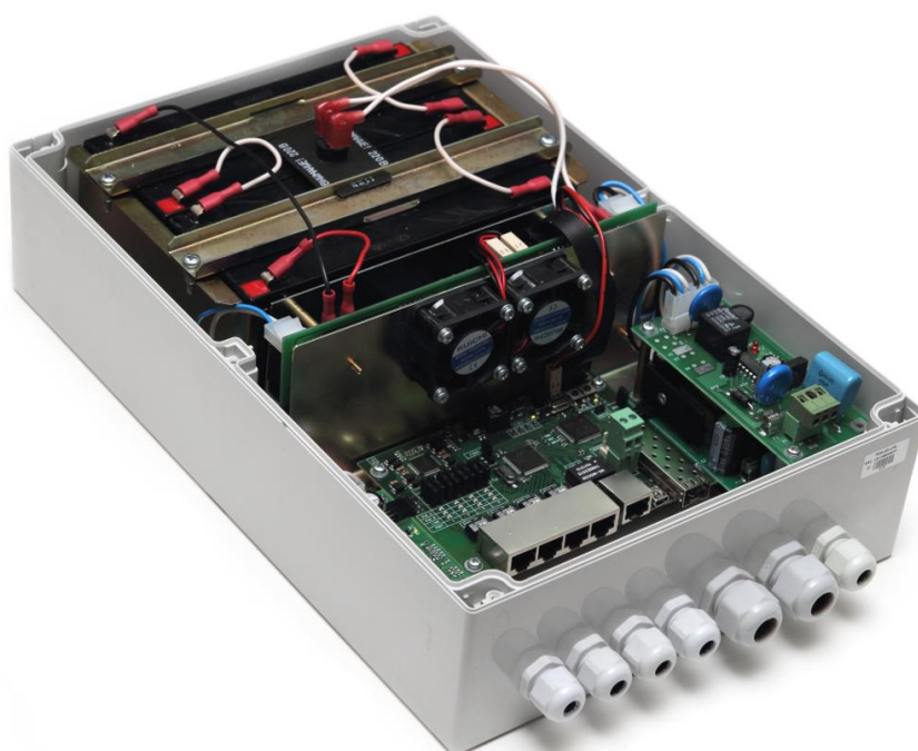
Рис. 2.1-5. PSW-1G4F-UPS - вид внутри
