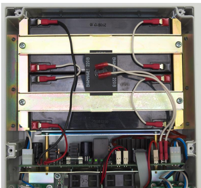
Рис. 2.9.5. Подключение АКБ.
