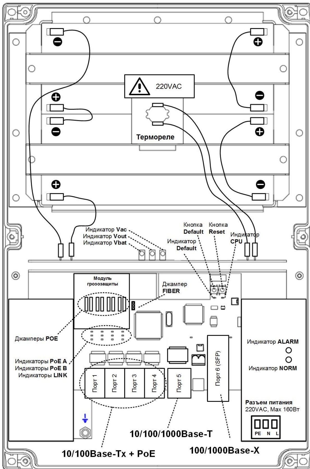
Рис. 2.2-2. Расположение элементов PSW -1G4F-UPS
