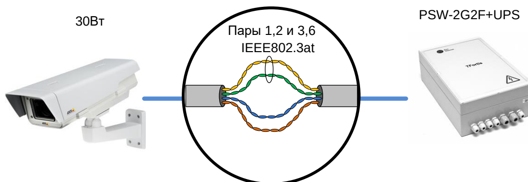
Рис. 2.3-2. Схема питания по PoE+ (30 Вт)
