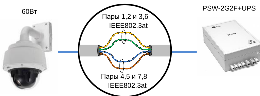
Рис. 2.3-1. Схема питания по PoE+ (60 Вт)
