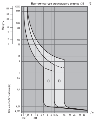
Рис. 1. Время-токовые характеристики
